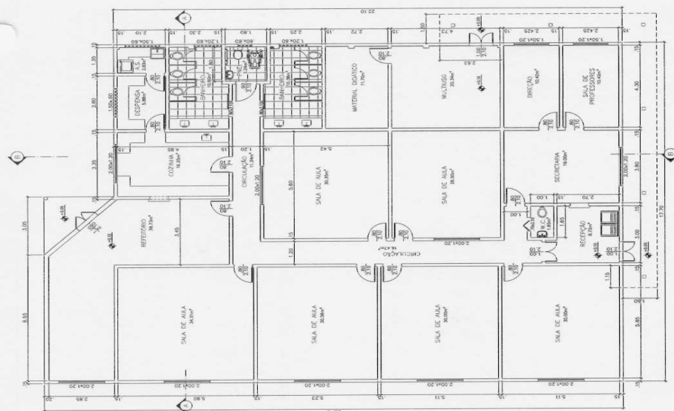
1 PLANTA BAIXA 6 ESCALA 1:75
